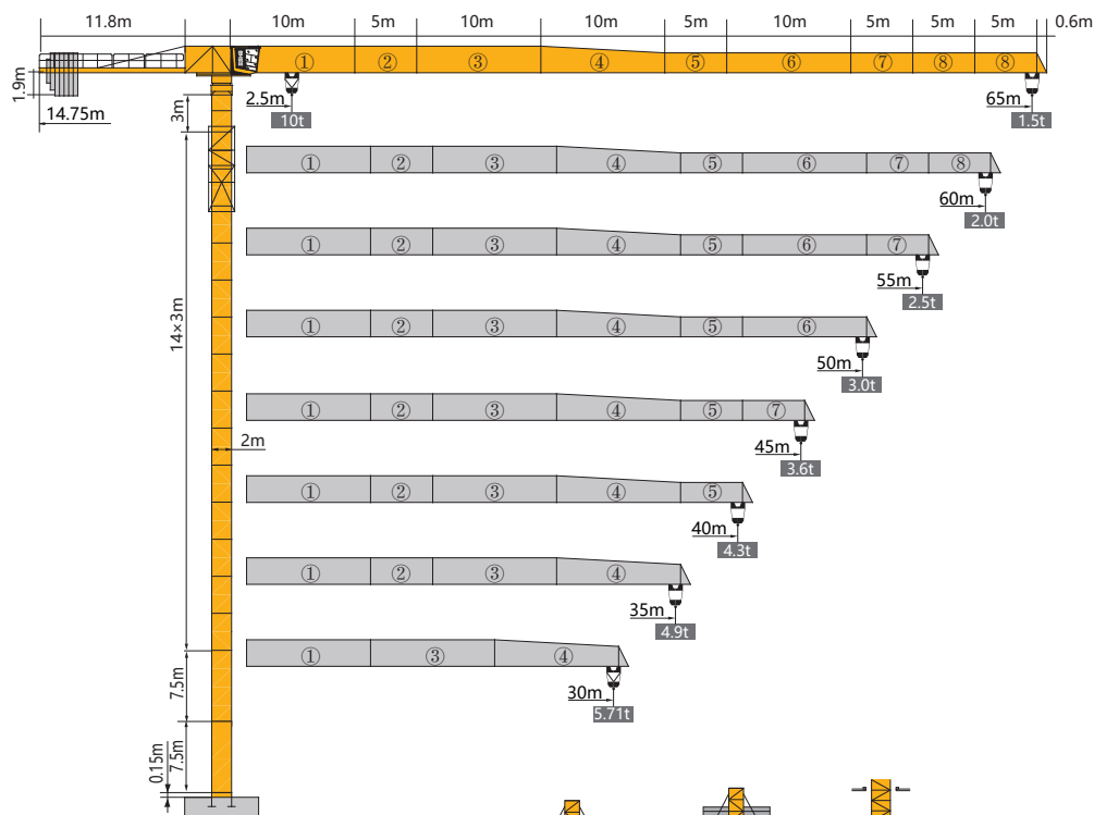
固定式 Stationary
