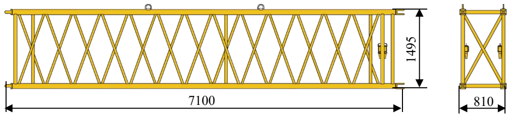
主臂加长节 618 kg Boom extension 618 kg
